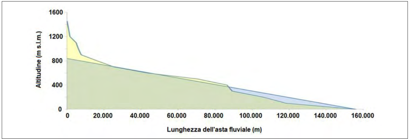
FIGURA 11. Sezione 1: pendenza media dell'asta principale i = 0,0073 (m/m), calcolata tramite il metodo grafico dell'area equivalente (Rif. WEB n. 7).
