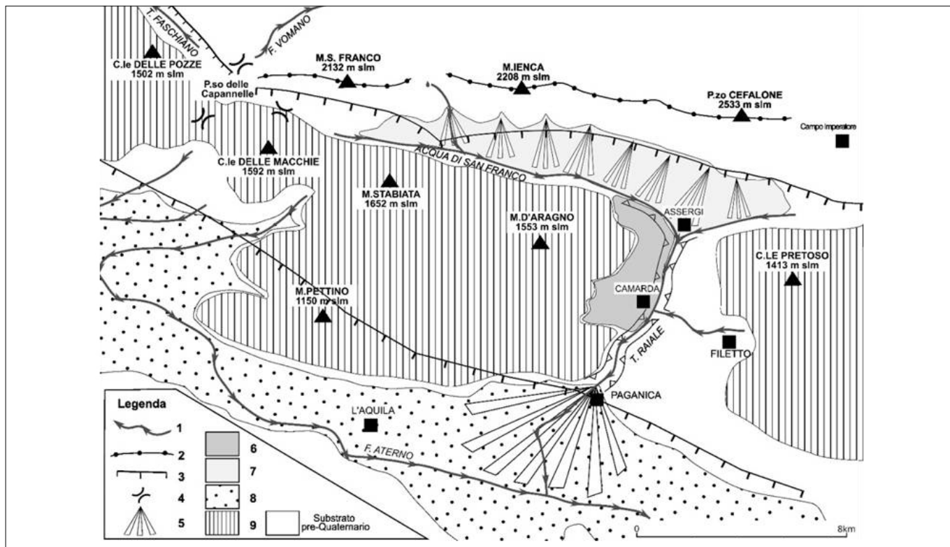
FIGURA 3. Schema geomorfologico dell'area del bacino del T. Raiale. 1. Corso d'acqua e direzione dello stesso; 2. Cresta; 3. Scarpa di faglia; 4. Sella o windgap; 5. Conoide alluvionale; 6. Depositi fluviali e fluvio-glaciali del Pleistocene Medio; 7. Depositi fluviali, fluvio-glaciali e di versante del Pleistocene Superiore-Olocene; 8. Depositi fluviali di fondovalle e terrazzati del Pleistocene Superiore-Olocene; 9. Forme Carsiche diffuse.
