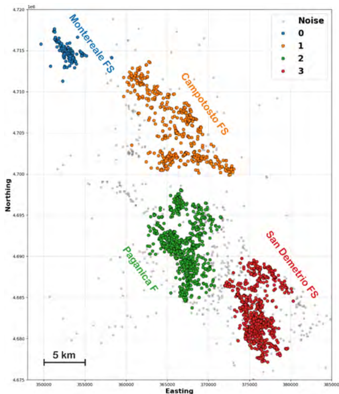
FIGURA 2. Mappa dei quattro cluster identificati dall'algorithm HDBSCAN con min\_samples=45 e min\_cluster\_size=45 . I cluster sono evidenziati con colori distinti: Montereale FS (blu), Campotosto FS (arancione), Paganica Fault (verde) e San Demetrio FS (rosso). I punti di noise sono visualizzati in grigio, indicando la loro appartenenza a nessun cluster significativo.
