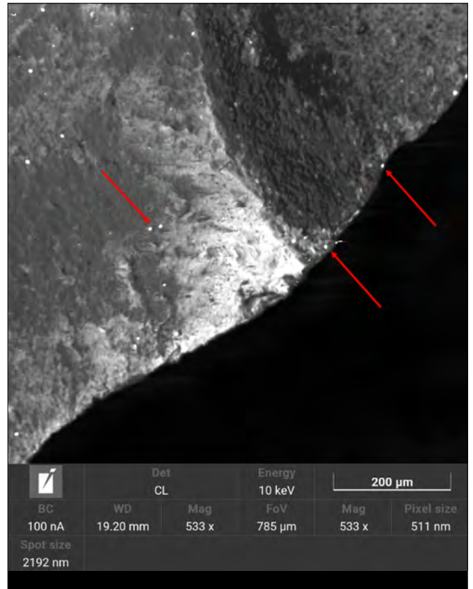
FIGURA 12. Immagine CL di una porzione di un frammento della frazione centimetrica del campione MB_1. Le frecce evidenziano gli spot che danno catodoluminescenza.
