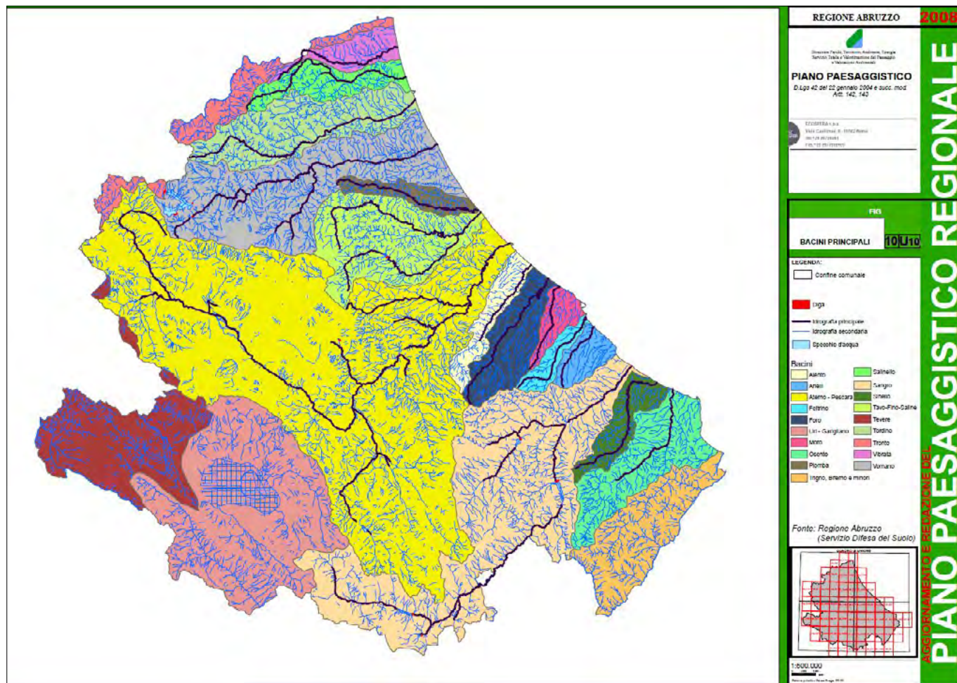
FIGURA 3. Piano Paesaggistico della Regione Abruzzo, tavola 10: Principali corsi d'acqua e relativi bacini idrografici.
