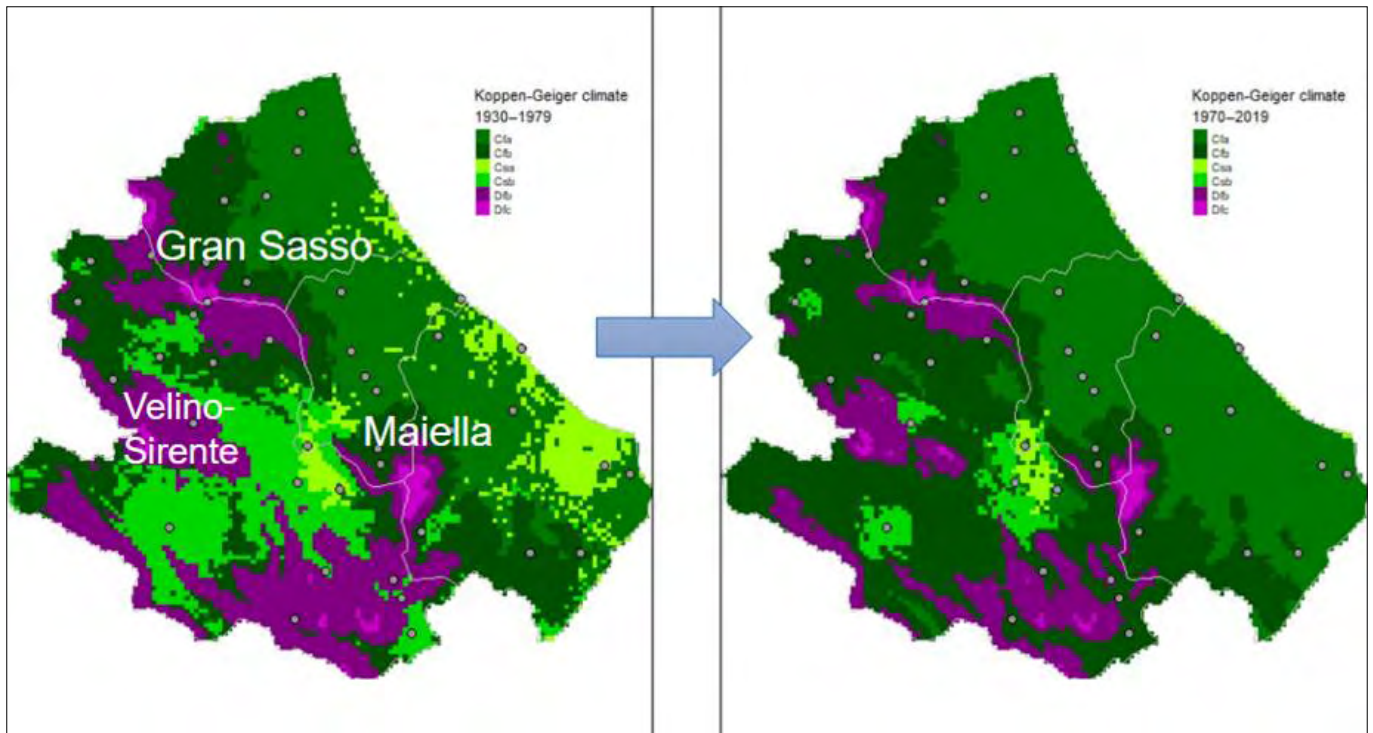
FIGURA 8. Classificazione di Koppen - Geiger (fonte: Curci et al. , 2021).
