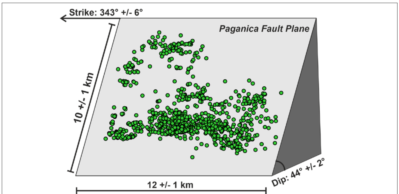
FIGURA 3. Schema della faglia di Paganica, attivata dal terremoto Mw 6.1 de L'Aquila. La figura mostra le dimensioni e l'orientamento della sorgente sismogenetica, così come calcolate in questo studio. In verde sono riportati gli ipocentri appartenenti al cluster 2, Paganica F, in Figura 2.
