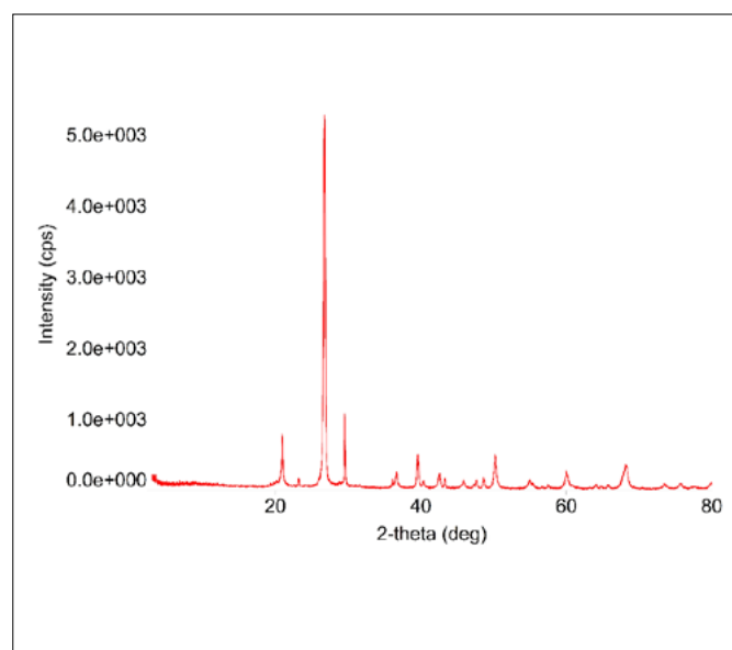
FIGURA 3. Diffrattogramma del campione MC_1.
