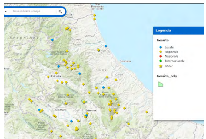
FIGURA 1. Inventario Nazionale dei Geositi Ispra: i geositi censiti per l'Abruzzo.
