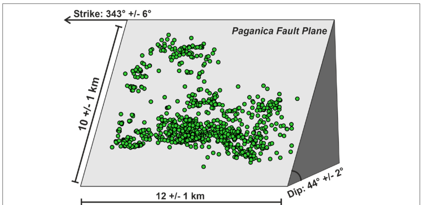
FIGURA 3. Schema della faglia di Paganica, attivata dal terremoto Mw 6.1 de L'Aquila. La figura mostra le dimensioni e l'orientazione della sorgente sismogenetica, così come calcolate in questo studio. In verde sono riportati gli ipocentri appartenenti al cluster 2, Paganica F, in Figura 2.
