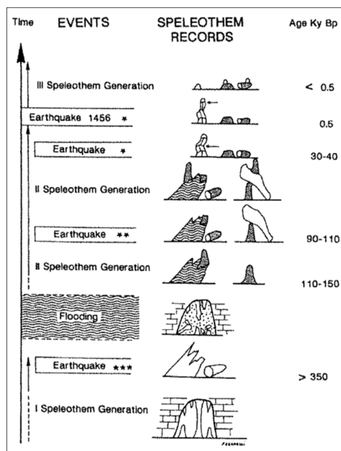
FIGURA 1. Evoluzione temporale delle fasi di concrezionamento e dei terremoti (da Postpischl et al. 1991).
