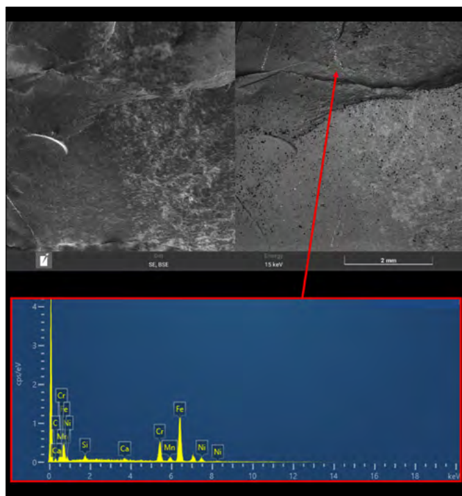
FIGURA 11. Immagini in SE (sinistra) e BSE (destra) di una porzione di un frammento della frazione centimetrica del campione MB_1. È riportato lo spettro chimico dello spot identificato dalla freccia rossa.
