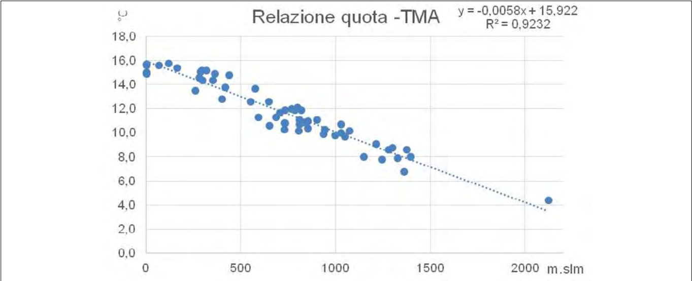
FIGURA 3. Relazione quota - temperatura media annuale (TMA).
