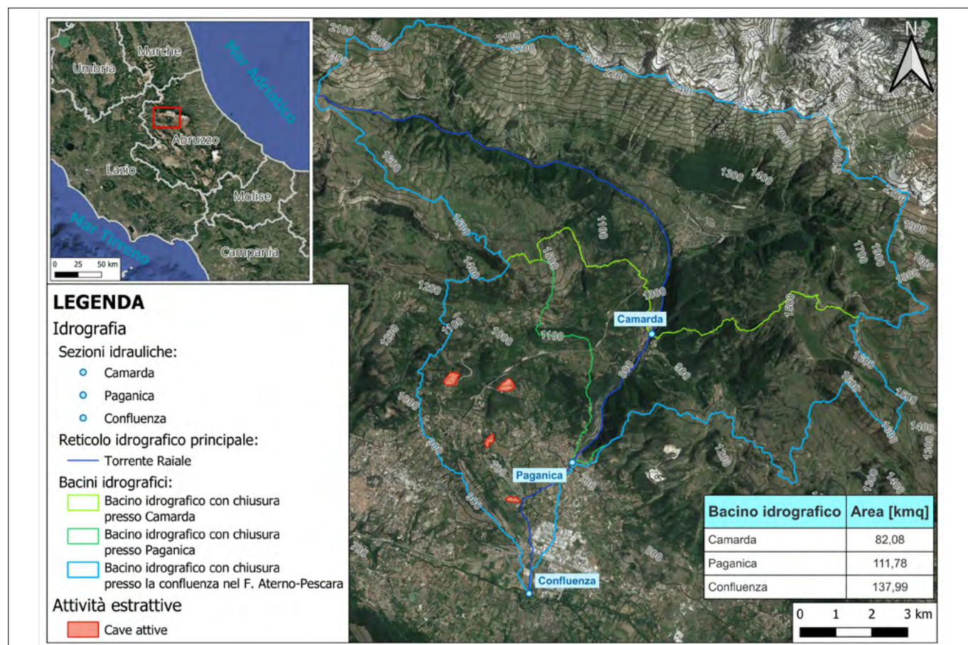
FIGURA 1. Ubicazione del bacino del T. Raiale. Nella figura vengono indicate le cave (cfr. par. 6) e le due sezioni fluviali analizzate (Paganica e Camarda), con i relativi bacini idrografici sottesi (cfr. par. 7).
