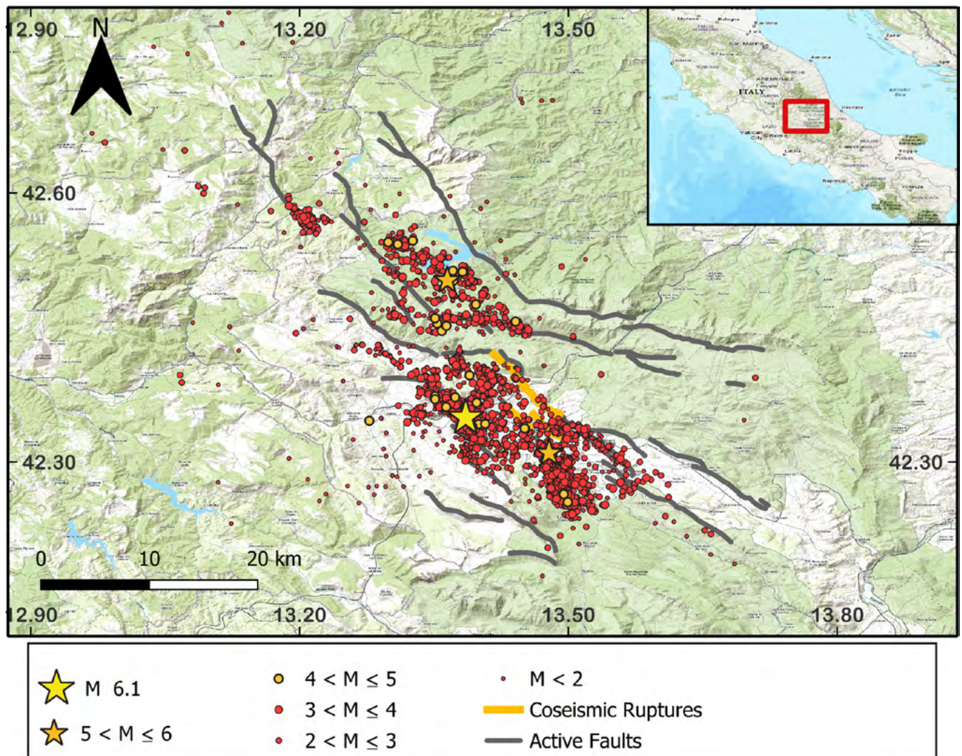
FIGURA 1. Mappa epicentrale della sequenza sismica de L'Aquila del 2009 (Mw 6.1), che mostra tutti i terremoti registrati da gennaio a dicembre 2009. La scossa principale è contrassegnata con una stella gialla, mentre le scosse di assestamento con Mw > 5 sono mostrate in arancione. I terremoti con magnitudo compresa tra 4 e 5 sono rappresentati da cerchi arancioni, mentre gli eventi più piccoli sono visualizzati in rosso, in scala di magnitudo. Le faglie attive e la traccia delle rotture cosismiche sono mappate secondo quanto riportato da LAVECCHIA et al. (2012). Le localizzazioni dei terremoti sono tratte da CHIARALUCE (2012).
