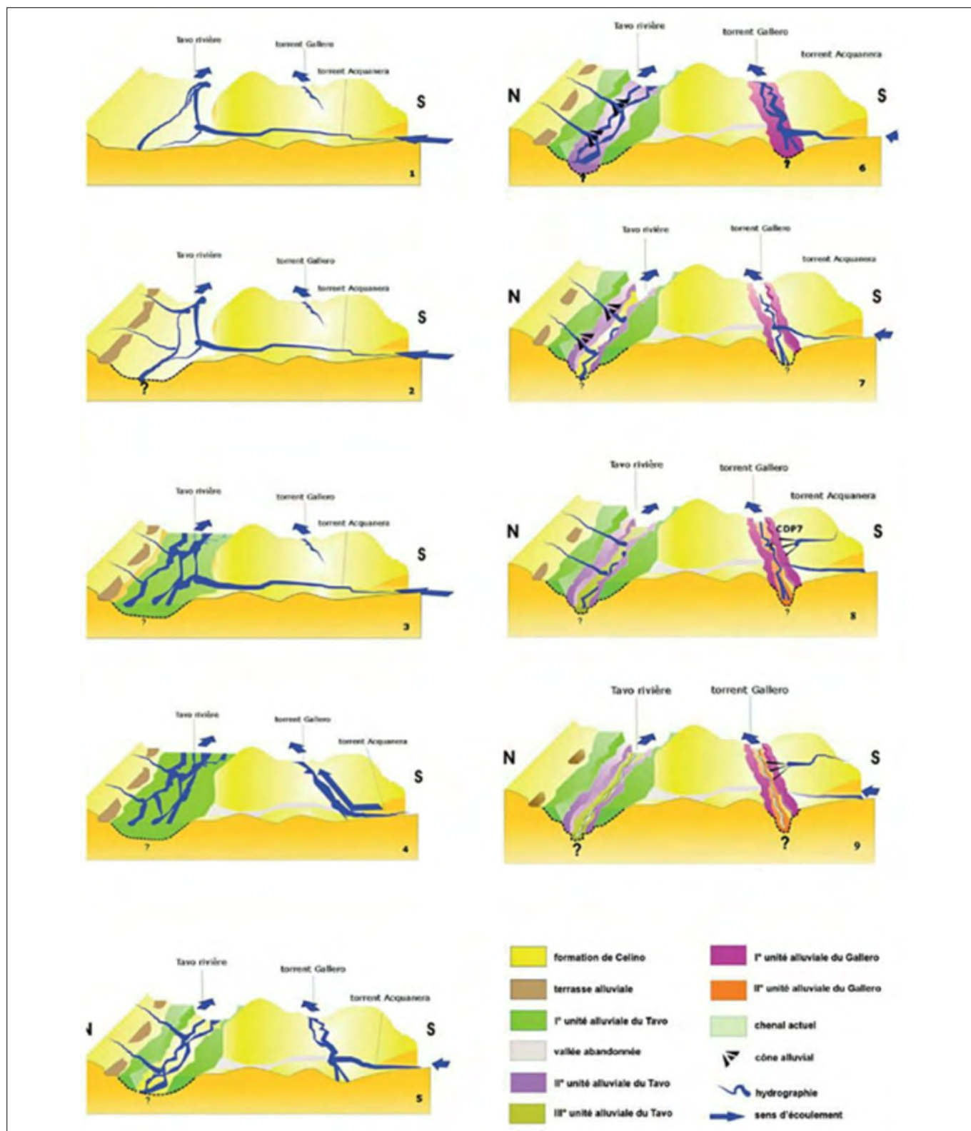
FIGURA 9. L'evoluzione del Fiume Tavo e del Torrente Gallero dal Pleistocene medio all'Olocene.
