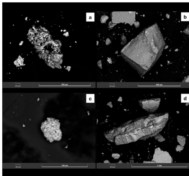
FIGURA 10. Immagini BSE della frazione millimetrica del campione MB_1: a) aggregato della frazione di granulometria millimetrica; b) frammento con granulometria millimetrica a spigoli vivi; c) frammento massivo con granulometria millimetrica con tracce di corrosione d); frammento con granulometria millimetrica di abito prismatico.
