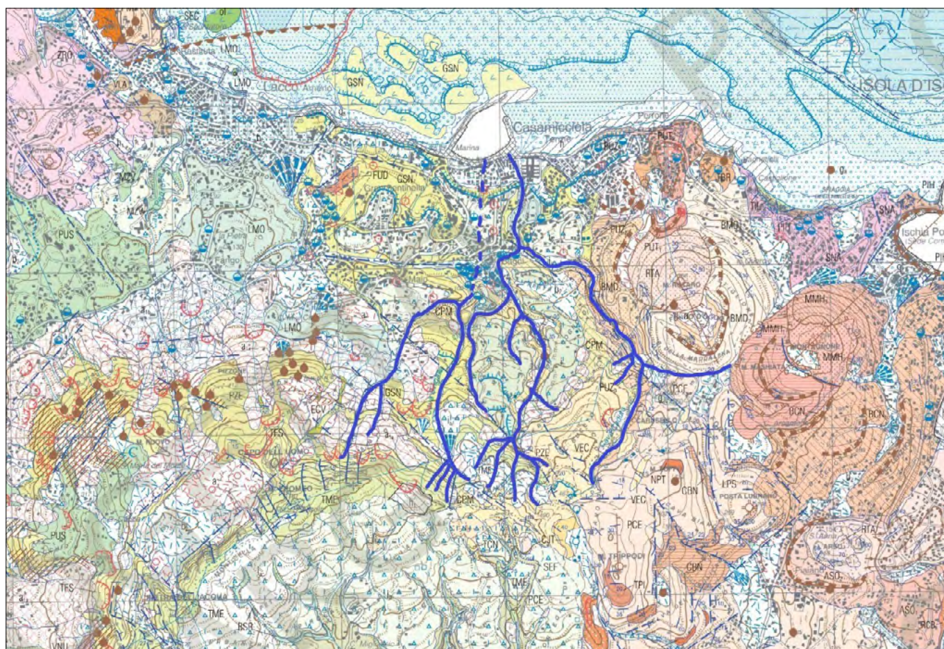
Figura 1. Reticolo idrografico sotteso al porto di Casamiccio su stralcio foglio Carg "464 - Isola d'Ischia"
