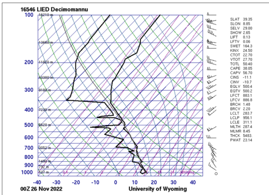
Figura 5. Diagramma skew-T relativo al radiosondaggio relativo alla stazione di Decimomannu (CA) effettuato alle ore 00 LT del 26 novembre
