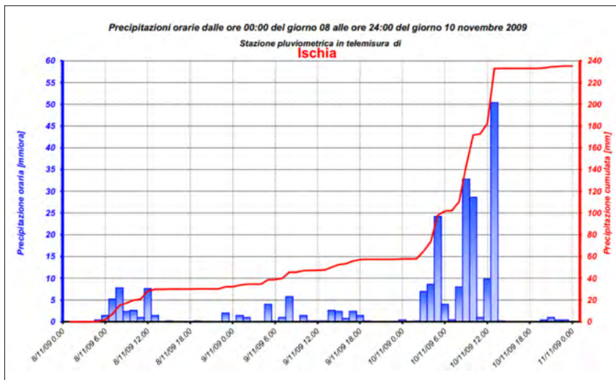
Figura 15. Precipitazioni orarie relative al timespan 00 AM del giorno 8 novembre 2009 alle 24 del giorno 10 novembre 2009 – pluviometro di Ischia porto (fonte CFR Campania)
