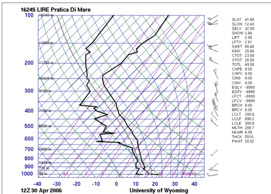
Figura 10. Diagramma termodinamico relativo alla stazione di Pratica di Mare alle ore 12 LT del 30 aprile 2006
