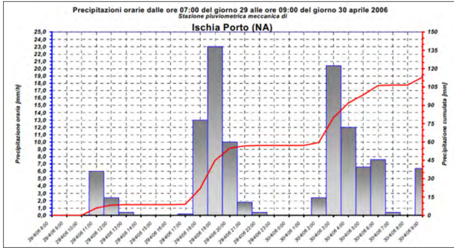
Figura 11. Precipitazioni orarie relative al timespan 7.00 AM del 29 aprile e le ore 9.00 AM del 30 aprile - pluviometro di Ischia porto (fonte CFR Campania)
