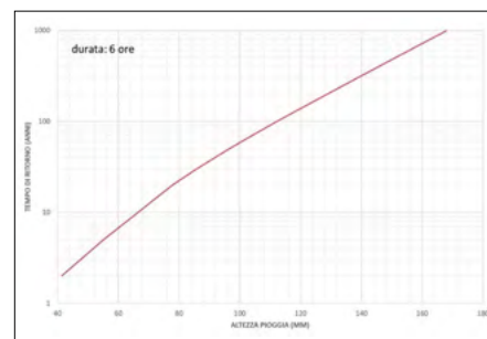
Figura 7. Stazione di Forio. Tempi di ritorno (TR) per pioggia di durata 6 ore con metodologia Valutazione delle Piene in Italia (VAPI)
