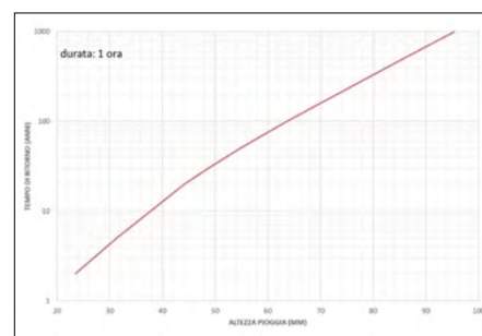
Figura 6. Stazione di Forio. Tempi di ritorno (TR) per pioggia di durata 1 ora con metodologia Valutazione delle Piene in Italia (VAPI)
